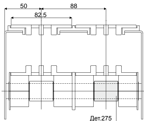
Пример установки
