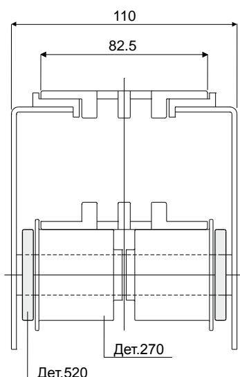
Дет.270
