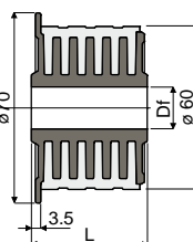
Type 1 (sans roulements)
