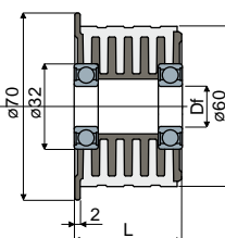
Type 2 (avec roulements)
