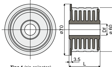
Tipo 1 (sin cojinetes)
