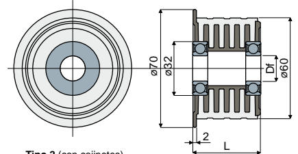
Tipo 2 (con cojinetes)
