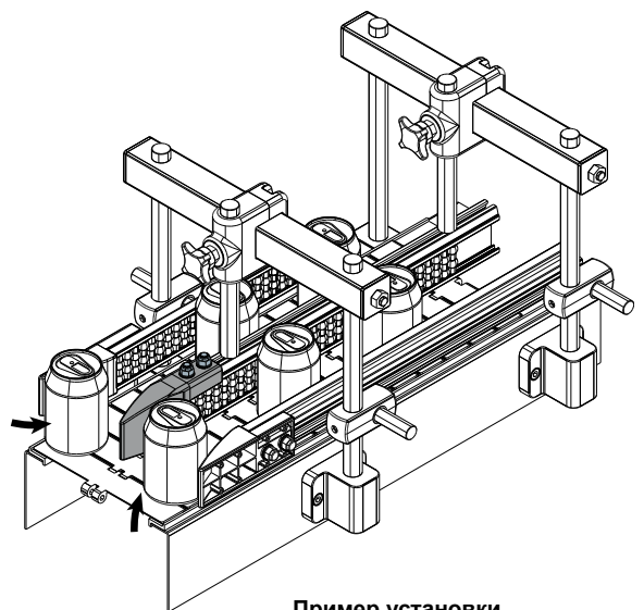
Пример установки
