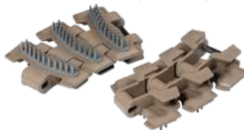
Криволинейная цепь с верхней резиновой частью (879 TAB BO)
