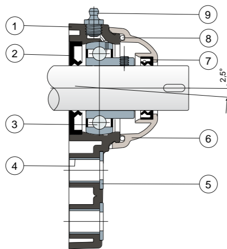
Полная защита подшипника
