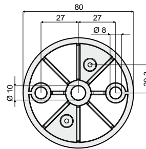
Ansicht von B (Distanzstück)
